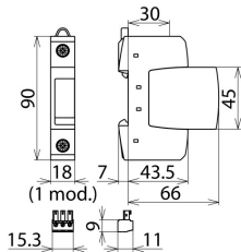
Dimension drawing DG SU 1P 120 R
